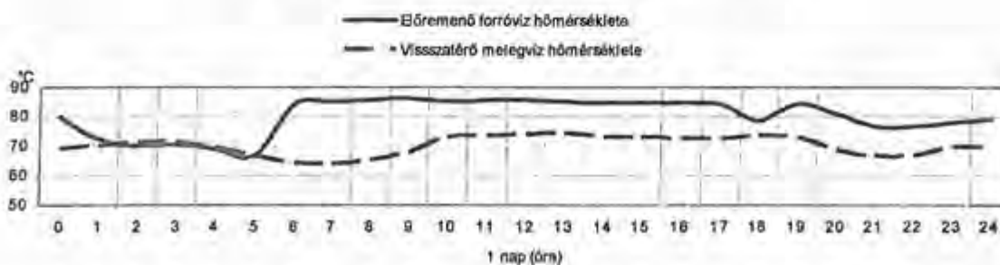
Primer előremenő és visszatérő forróvíz-melegvíz hőmérséklete
