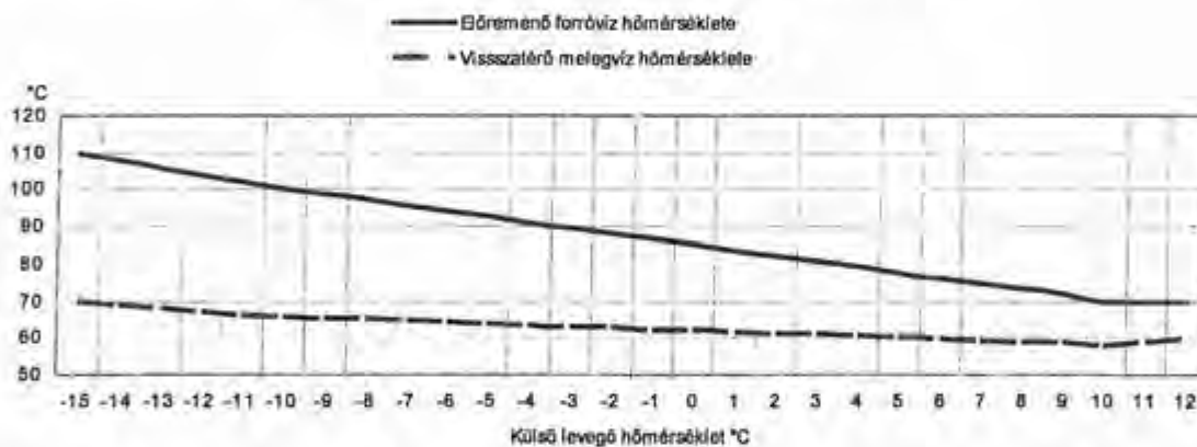
Primer előremenő és visszatérő forróvíz-melegvíz hőmérséklete
